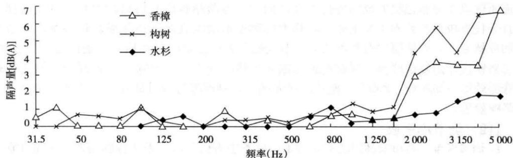
图 1-1-2 不同叶形树种隔声量比较 (郑思俊, 2006)
