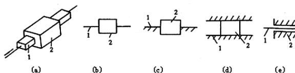
图 2 移动副及表示符号
